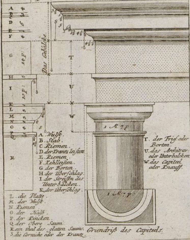
Toscanisches Capiteel und Gebälcke. 10.
