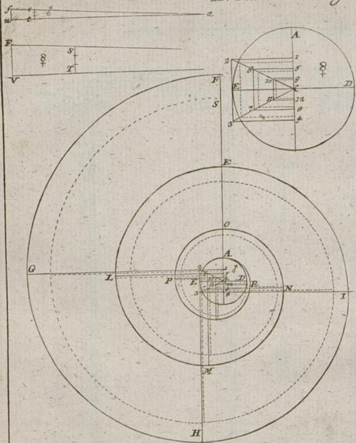
Aufreiffung der Goldmannischen Schnecken Linie. 25
