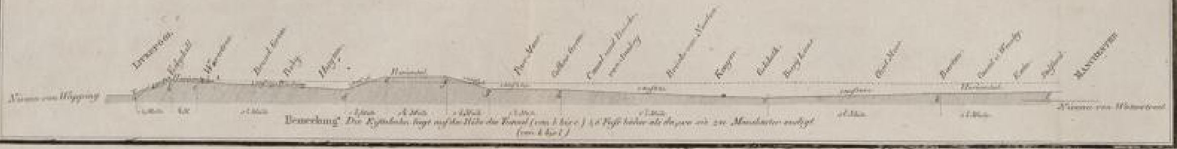
Profil der Eisenbahn zwischen Liverpool und Manchester.
