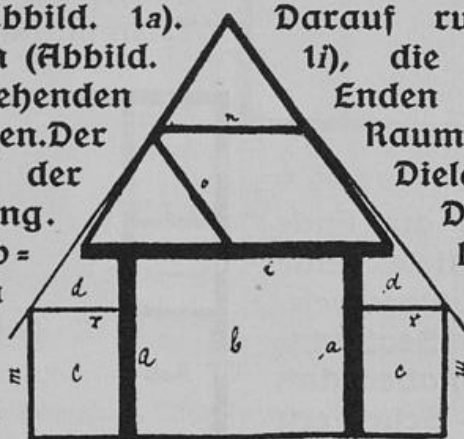
Abbild. 1. Querschnitt.
