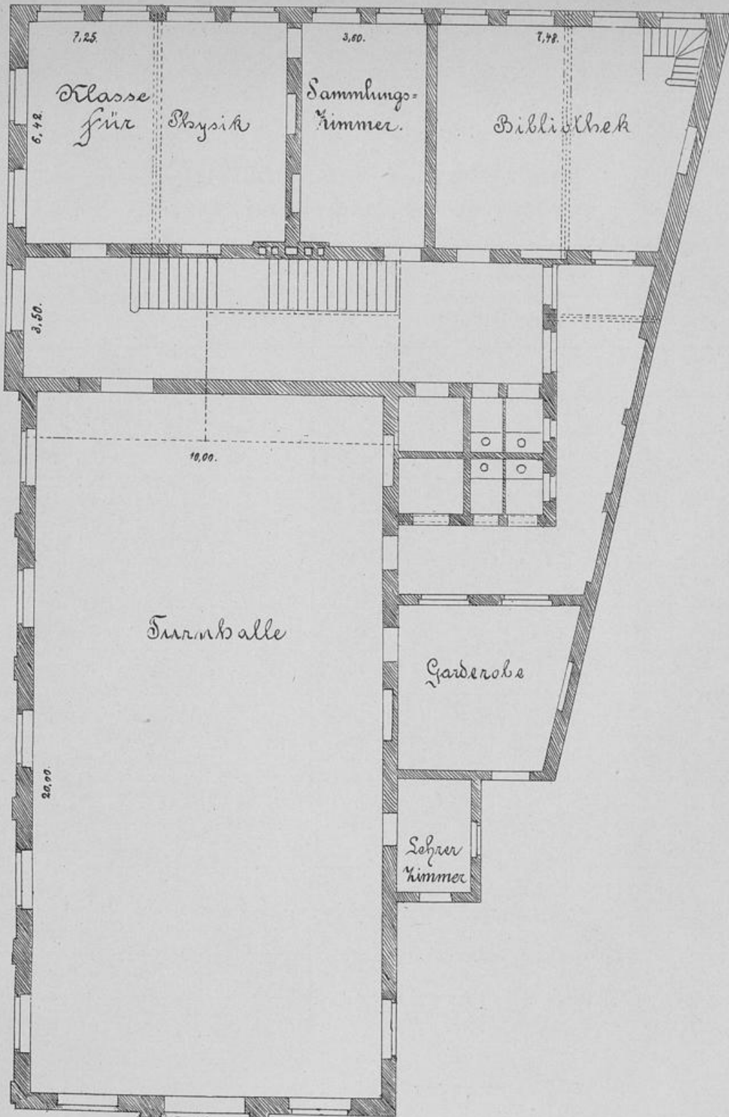
Grundriss des Erweiterungsbaues.
