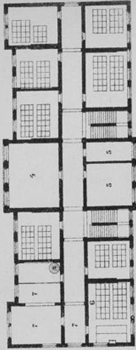
Erstes Obergeschofs.
