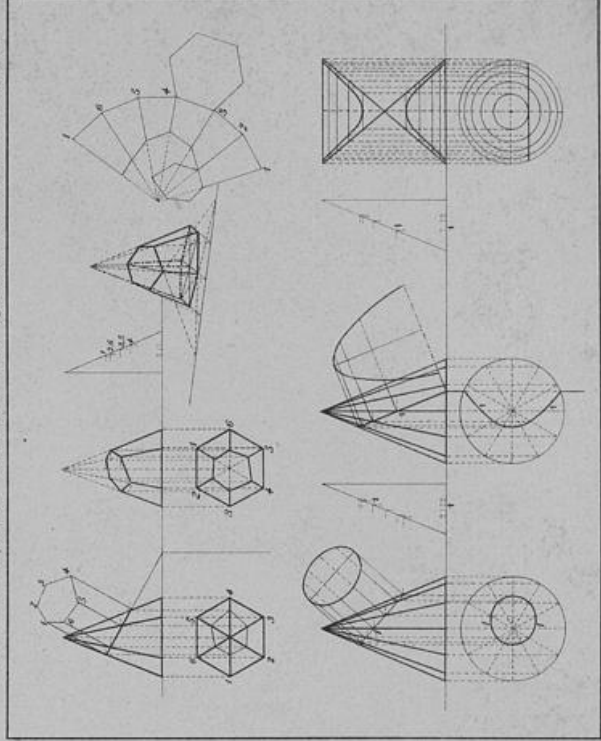
Blatt 14. Schiefe Schnitte der Pyramide und des Kegels.
