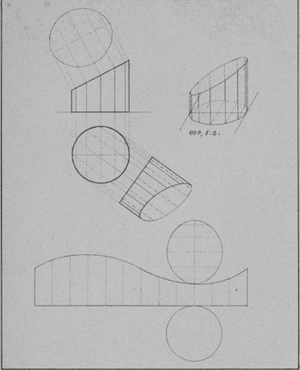
Blatt 13. Schiefer Schnitt des Cylinders.
