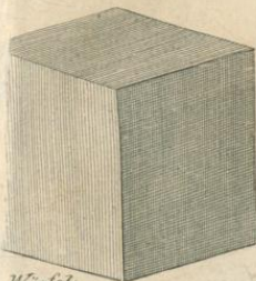
Würfel
