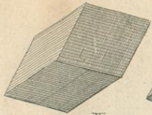
Rhomboeder X
