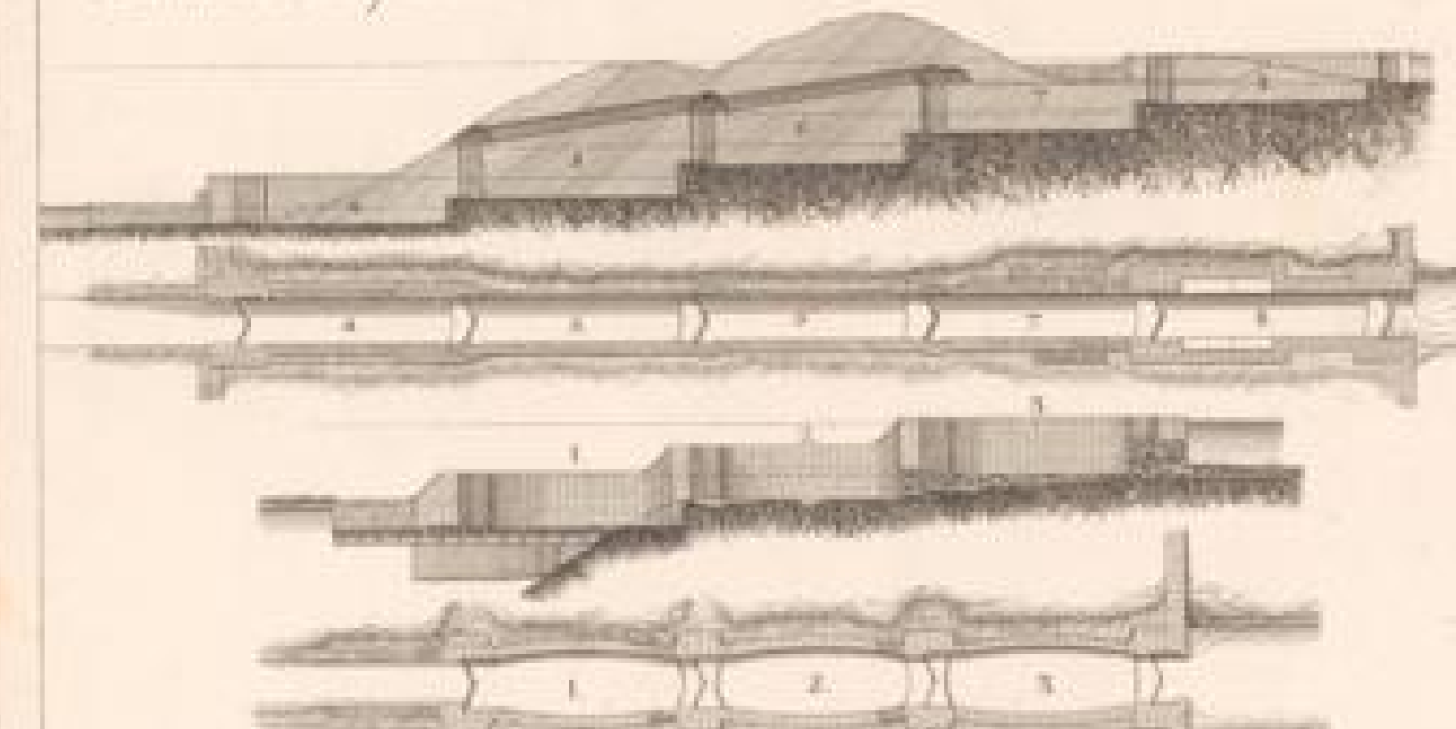
Profil Canal de Castagnon
