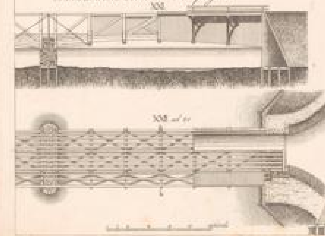
Profil Canal en bois sur page 33
