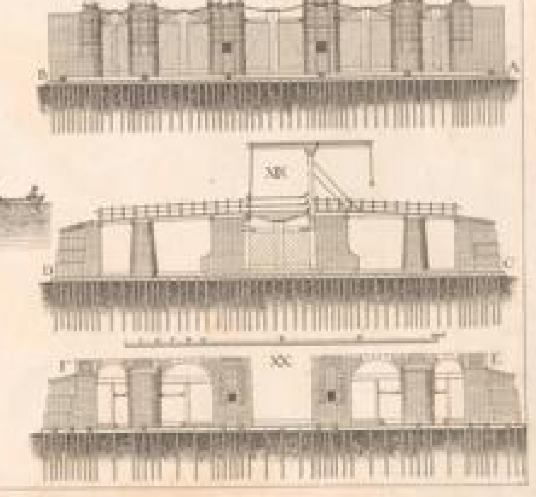
Élévation de l'écluse de Mayden sur la Côte de la Mer
