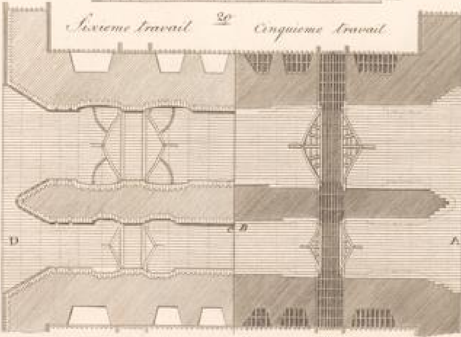
Ecluse de Gravellines de 1699
