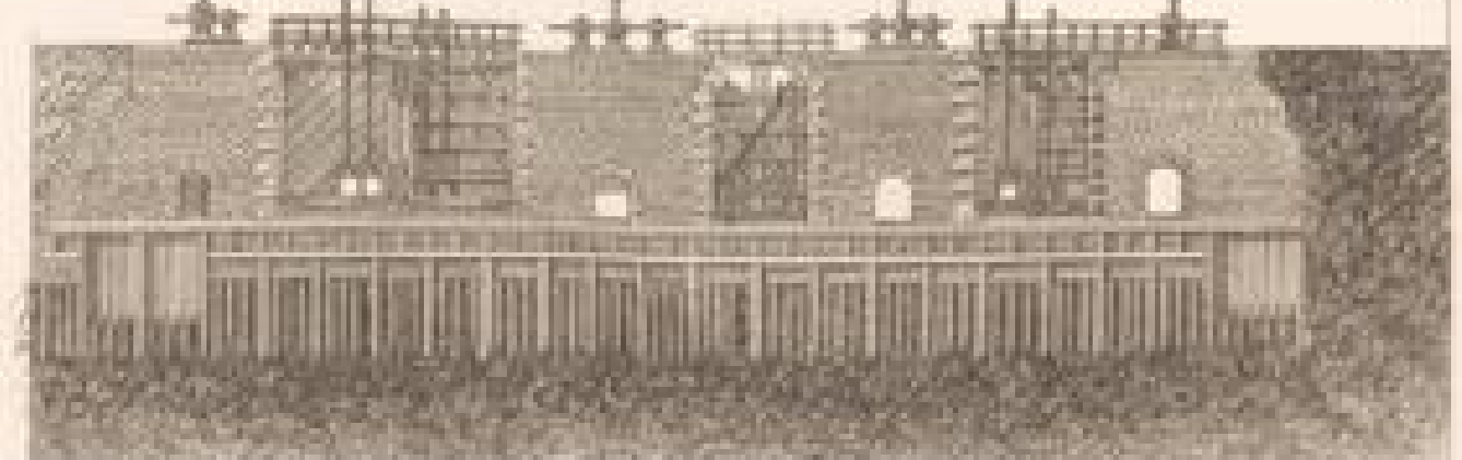
Coupe sur la Ligne y h i k l m n o p q r s Tab 73
