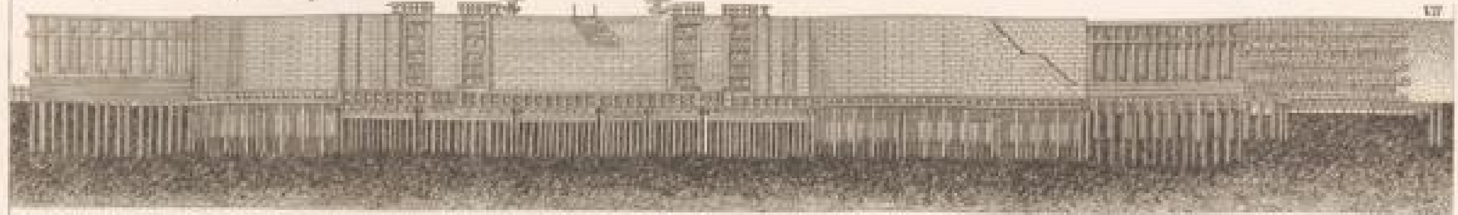
Coupe & Elevation sur la Ligne i k l m n o Tab 73
