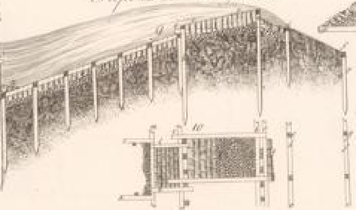
Profil des Seufsbau bei Ostende
