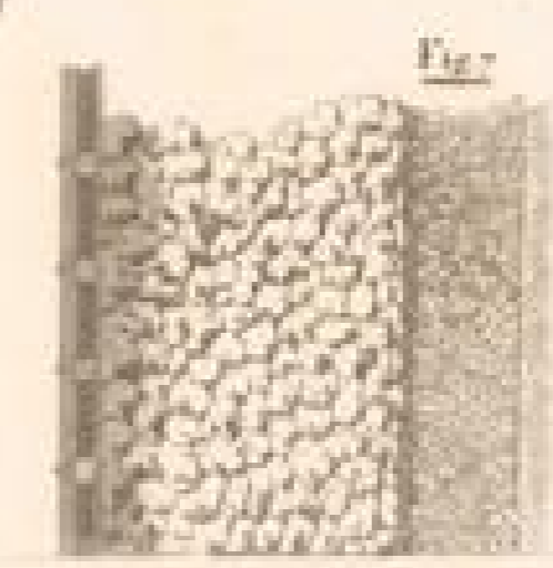
Horizontaler Durchschnitt und obere Lage eines MOLEN zur Einfahrt und Sicherung eines Seehafens, so zur Erhaltung des Meerufers
