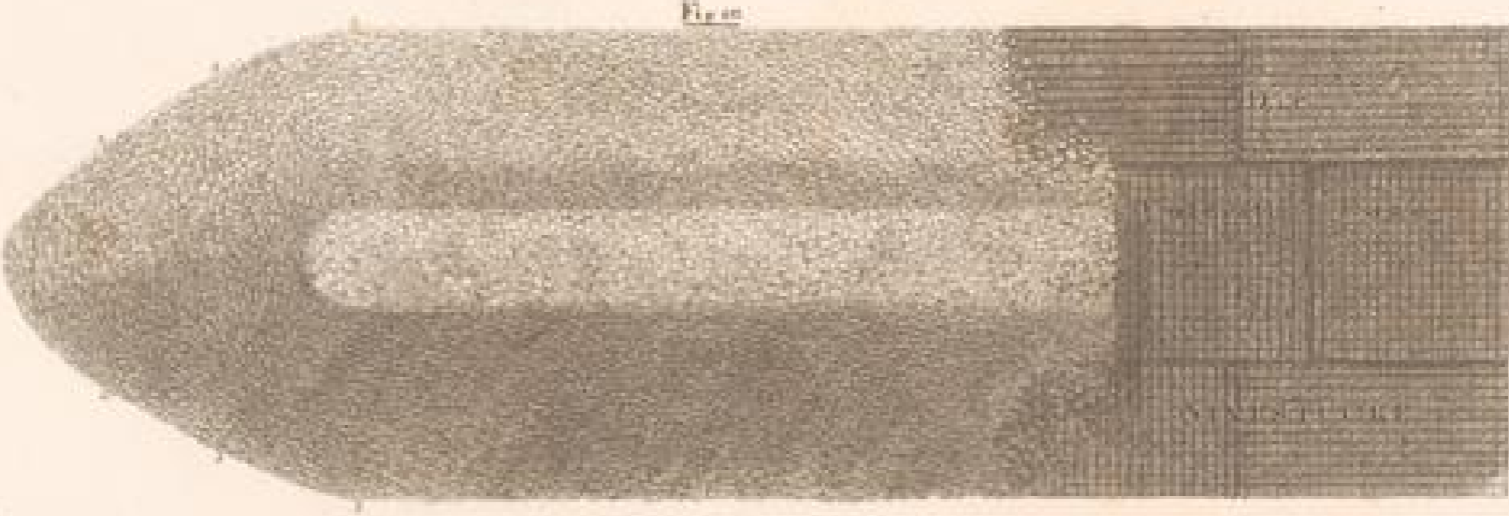
Horizontaler Durchschnitt und obere Lage eines MOLEN zur Einfahrt und Sicherung eines Seehafens, so zur Erhaltung des Meerufers
