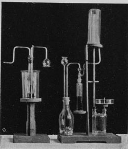
Abbildungen zu Erb: Apparate für chemischen Experimentalunterricht.
