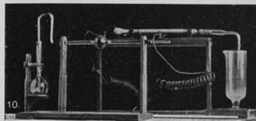
Abbildungen zu Erb: Apparate für chemischen Experimentalunterricht.
