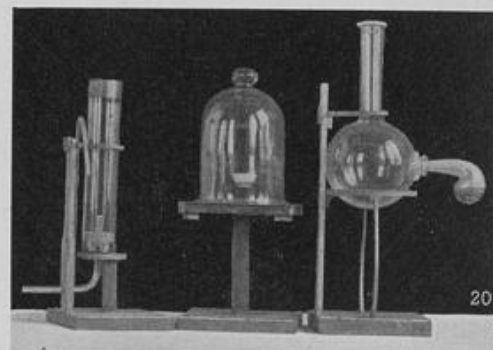
Abbildungen zu Erb: Apparate für chemischen Experimentalunterricht.
