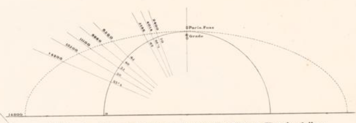
Höhe der Schneegränze in der nördlichen Hemisphäre (nach Alex. Freyh. von Humboldt.)
