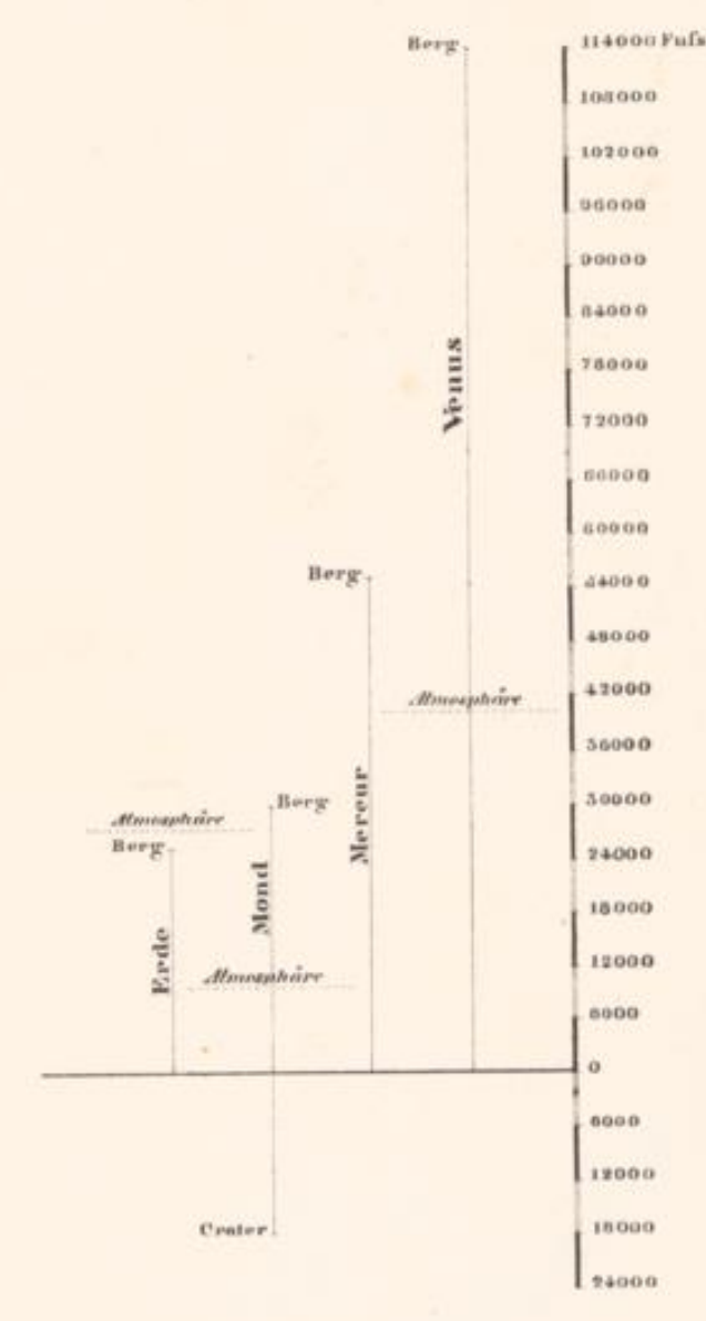
Verhältnisse der Berge und Atmosphären auf mehreren Planeten (nach Tobias Mayer.)
