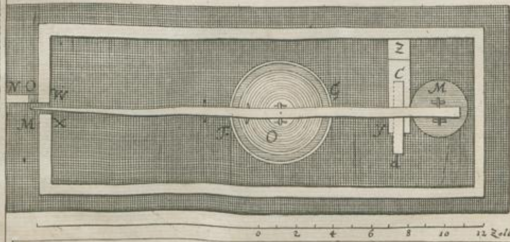
Hydrostatische waage des Hrn. Ingenieur Hauptm. Cassens
