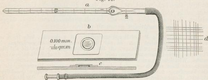
Blutkörperchenzählapparat nach Thoma-Zeiss.
