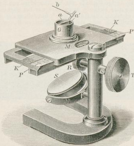
Hämometer von Fleischl.
