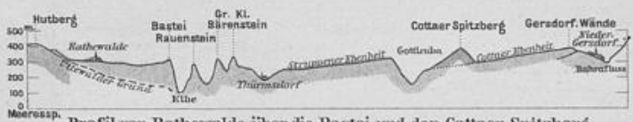
Profil von Rathewalde über die Bastei und den Cottaer Spitzberg nach Nieder-Gersdorf.
