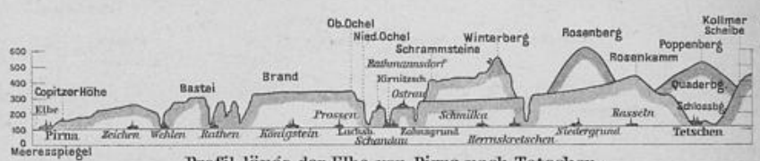
Profil längs der Elbe von Pirna nach Tetschen. Maßstab der Länge 1: 400.000, M. d. Höhe 1: 40.000.
