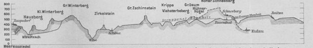
Profil von Saupsdorf über die Winterberge, den Gr. Zschirnstein u. den Schneeberg nach Raitza.
