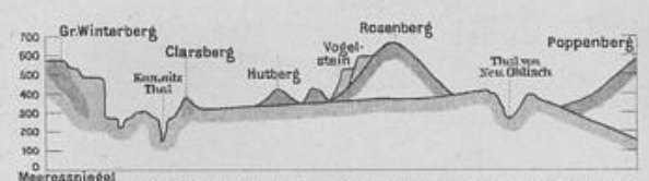
Profil vom Winterberg über den Rosenberg zum Poppenberg.
