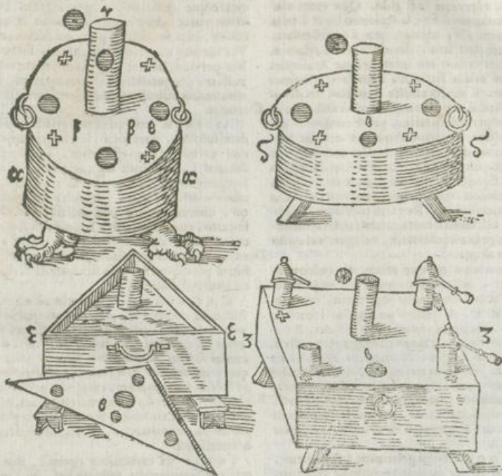
α. Vas balnei Mariae cupreum, resudum. ββ. Operculum rotundi vasis, cum quatuor foraminibus, per quæ cucurbitarum colla transiunt. γ. Canalis cum operculo perforato, & craticula in fundo. δ. A. Balneum oblongum pro duabus bocciis. ε. Balneum triangulare pro tribus bocciis. ζζ. Balneum quadratum pro quatuor bocciis. θ. Foramen, per quod aqua infunditur.
