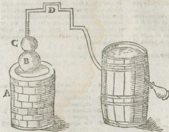
Fornax cum retorta.
