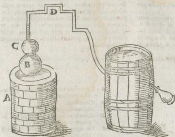
Fornax cum retorta.
