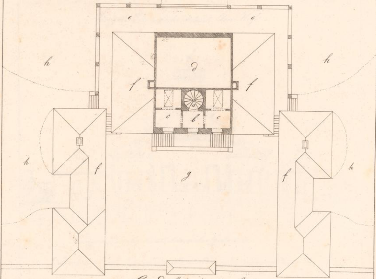
Grundriß des zweiten Stockes.
