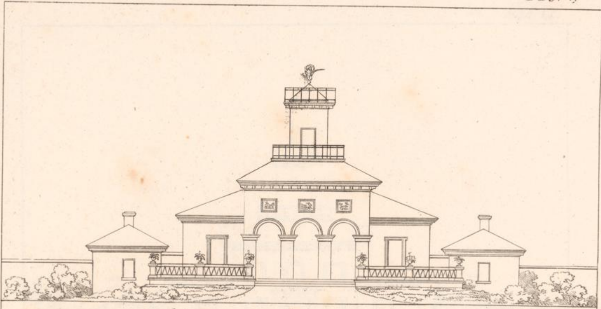
Aufsicht gegen den Garten auf die Ostseite.
