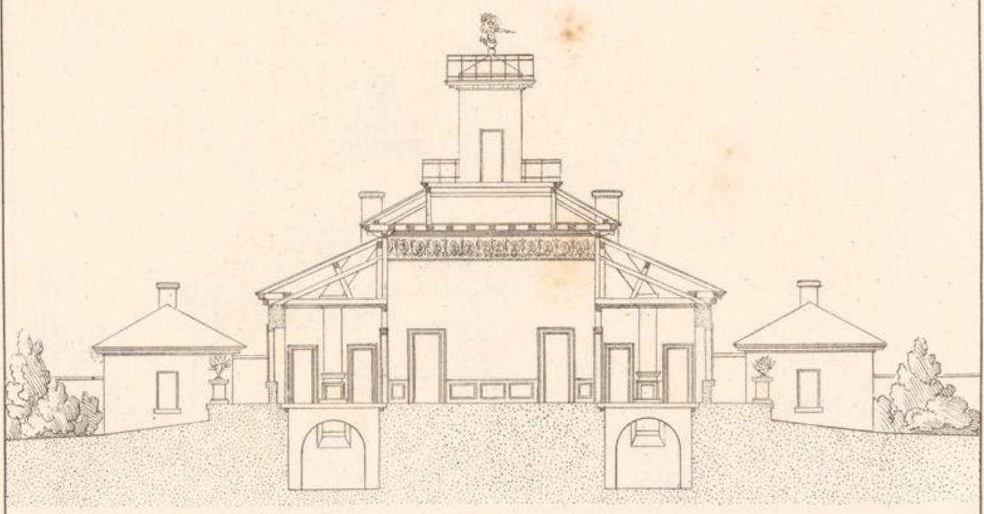
Längen Durchschnitt durch das Gebäude
