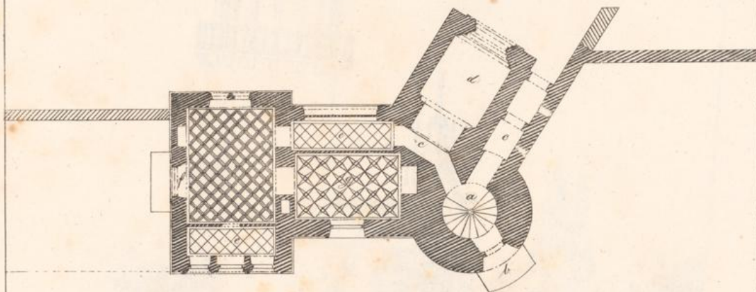
Grundriß des 2 ten Stock.
