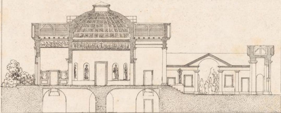
Querdurchschnitt mit dem Eingang und der Ansicht des Hofes
