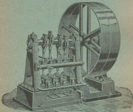
Hydraulische Presspumpe P. V.
