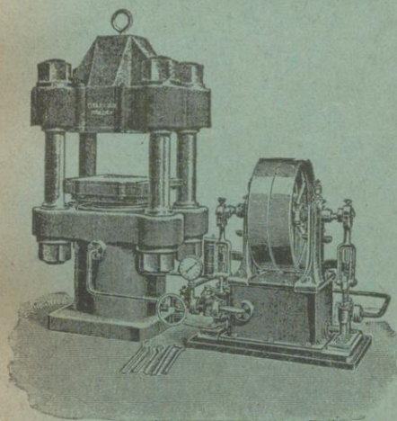
Hydraul. Presse H. P. 500.
