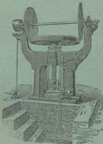
Spindelpresse S. P. V. 160.
