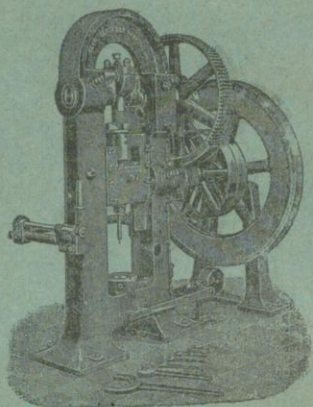
Tubenpresse T. P. III.
