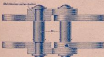
Gall'sche Union-Büchsen-Kette.
