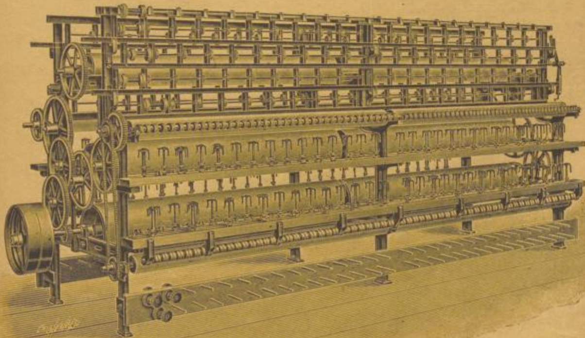
Gummiumspinnmaschine für einfache und Kreuzumspinnung mit neuer Gummifadenspannvorrichtung D. R. M. G.
