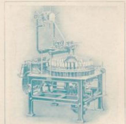
Einfädige Spitzenmaschine für sogenannte Handklöppelspitzen
