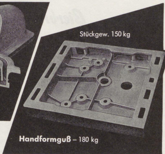
Sandguß maschinengeformt
