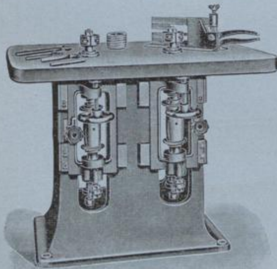
Tischfräsmaschine.
