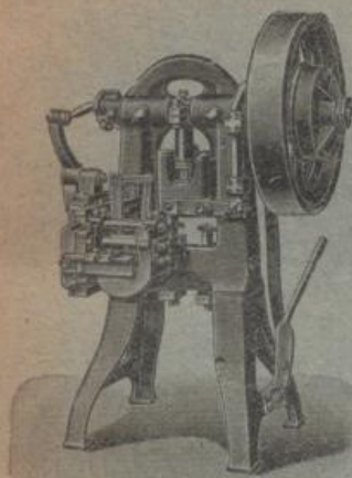
Autom. Presse mit Richtmaschine.
