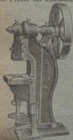
Einarm. Exzenterpresse
