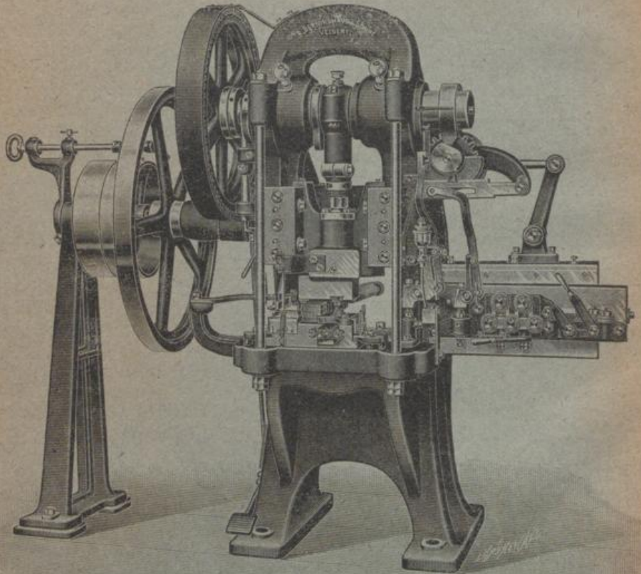
Hangschloss-Bügelautomat (30 Stück fertige Bügel per Minute).
