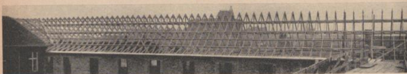
VOLLMAR-BOHLEN-DACH-KONSTRUKTION HAUPTVERWALTUNGSGEBAUDE DER LANDESVERSICHERUNGSANSTALT FÜR NORDRHEIN-WESTFALEN IN DÜSSELDORF AUSGEFÜHRT 1949
