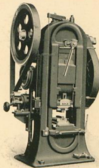
Kniehebel-Prägepresse
