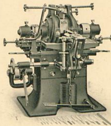
Messerschleifmaschine
